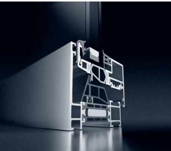
Ventana Schüco AWS 70 BS.HI Schüco Window AWS 70 BS.HI
