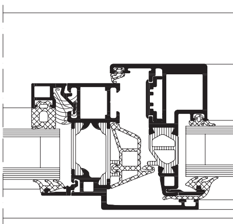
Detalle de una ventana flotante Escala 1:2 Detail of floating window Scale 1:2
