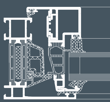
Ventana Schüco AWS 75 BS.HI Escala 1:2 Schüco Window AWS 75 BS.HI Scale 1:2
